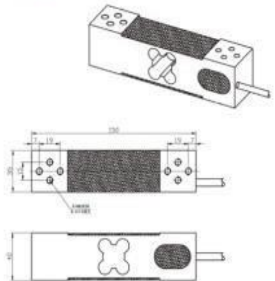
尺寸圖
